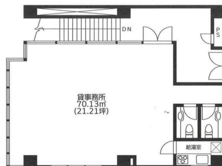
【平面図】
