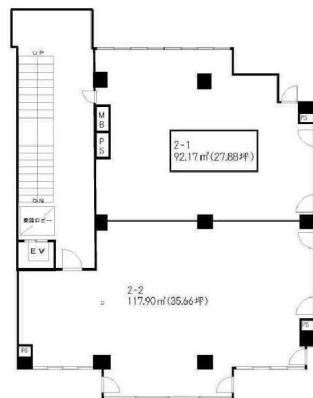
【平面図】
