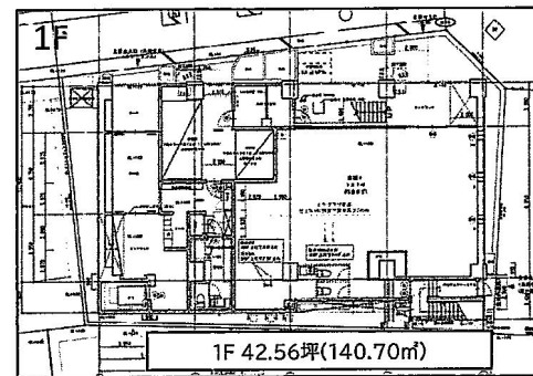
【平面図】
