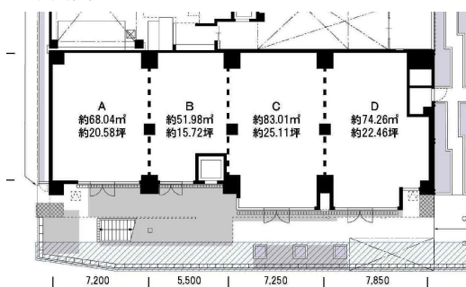
【平面图】
