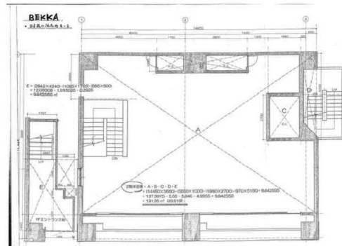
【平面図】
