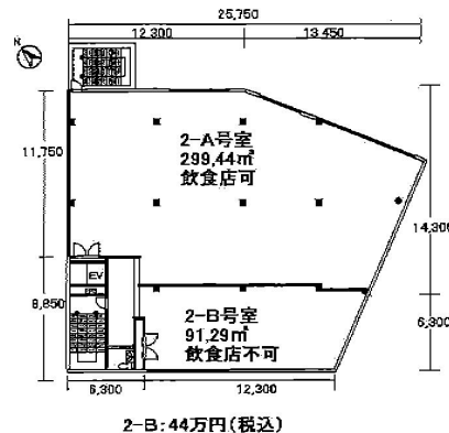
【平面図】
