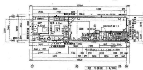
【平面図】
