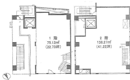
【平面図】
