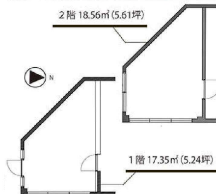
【平面图】
