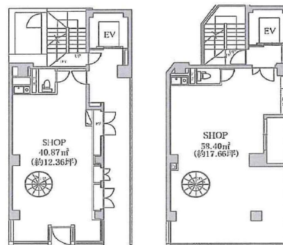
【平面図】
