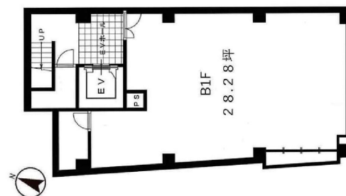
【平面図】
