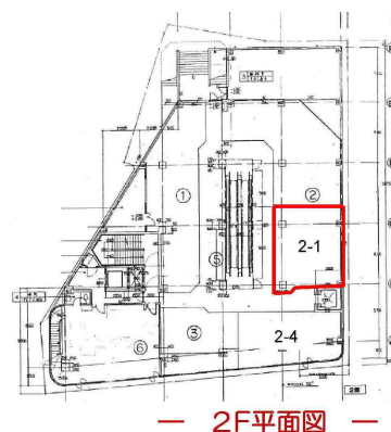
【平面図】
