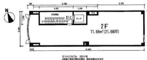
【平面図】
