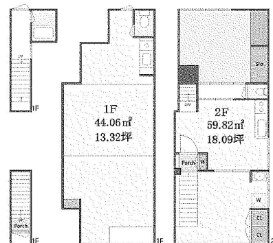
【平面図】
