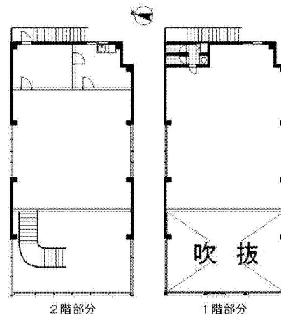
【平面図】
